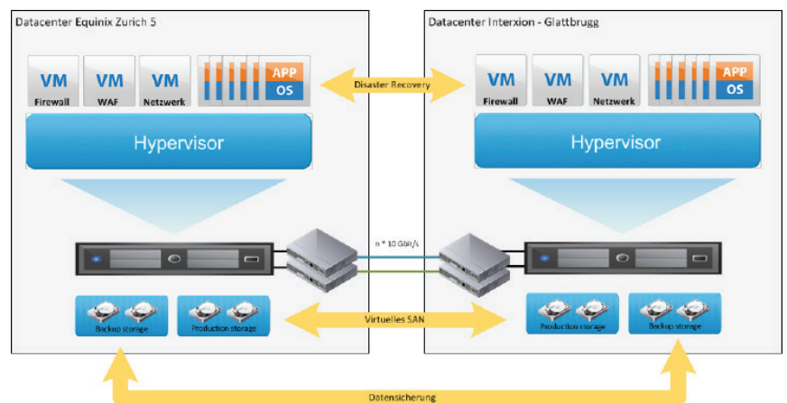
Aufbau der Virtual Private Cloud georedundant über zwei TIER-3 Datacenter.
